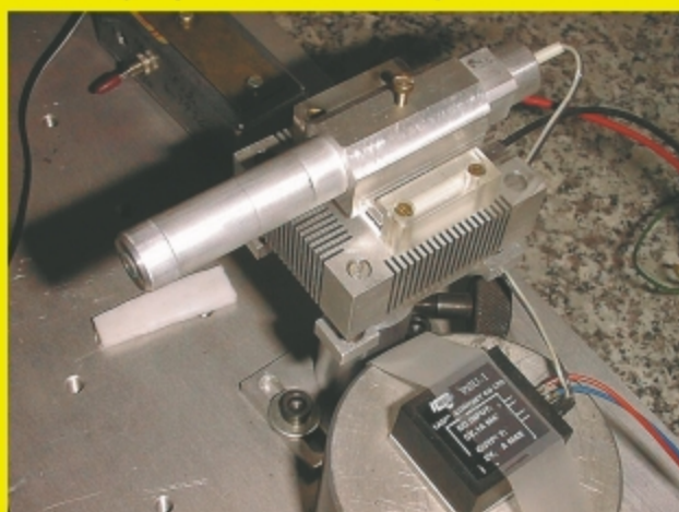
Mikrolaser neodymowy
